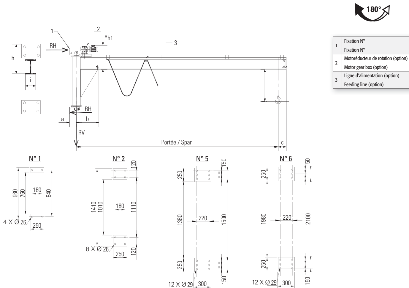
Détail des fixations / Fixation information
