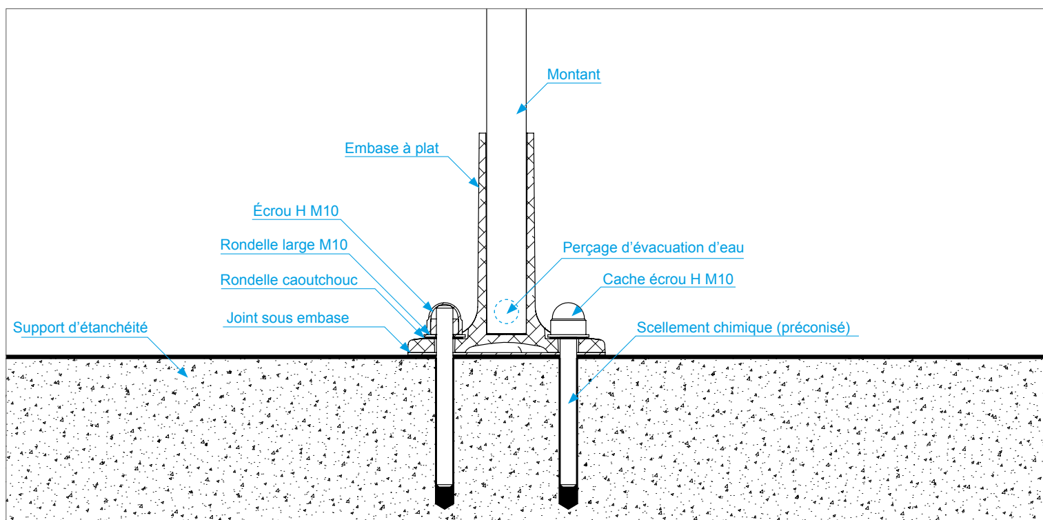
Joint et cache écrou
